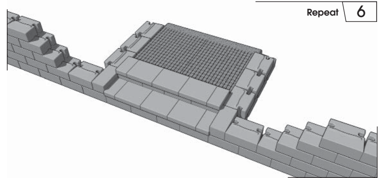
Geogrid Layer 4
